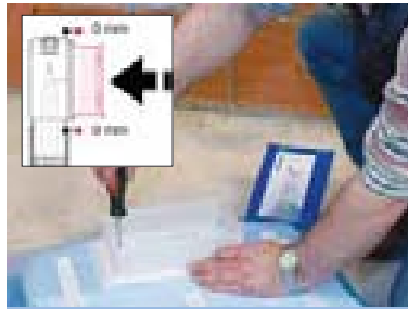
Montaggio della protezione cantiere
