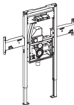
Modulo d'installazione per lavabo, parete altezza parziale.
