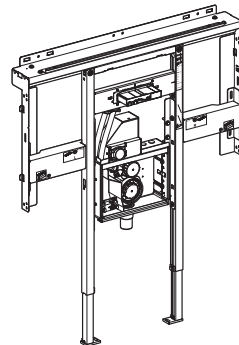
Modulo d'installazione per lavabo, parete altezza totale.
