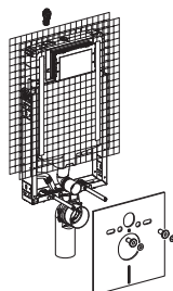
Combifix Sigma8 110.790.00.1 110.791.00.1
