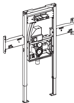
Modulo d'installazione per lavabo, parete altezza parziale.
