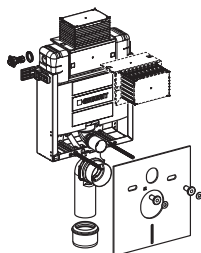
Combifix 90 Omega 110.000.00.1
