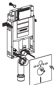
Combifix Sigma12 110.307.00.5 110.308.00.5
