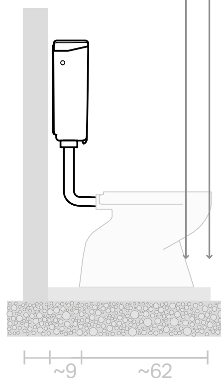
Confronto Geberit Combifix Sigma8 davanti alla parete e cassetta esterna.
