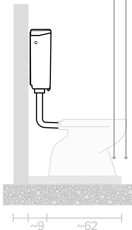
Confronto cassetta da incasso Geberit Sigma8 e cassetta esterna.
