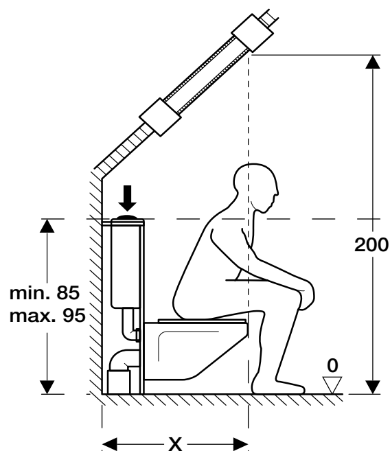
Combifix Omega o Duofix Omega per WC sospeso con attivazione del risciacquo dall'alto.
