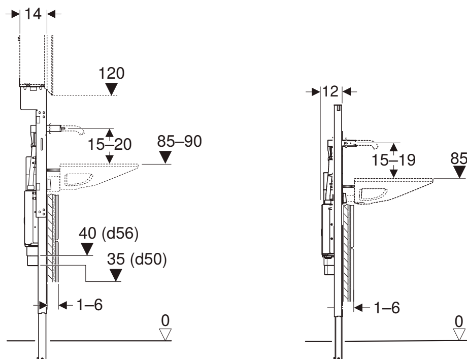
Figura 17: Parete leggera ad altezza totale e ad altezza parziale con elemento Geberit Duofix per lavabo
