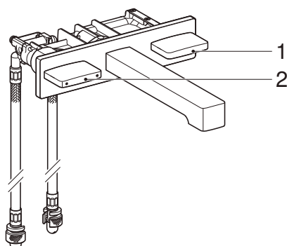
Figura 4: Rubinetteria, design squadrato, montaggio a parete, miscelatore a due manopole, per vano sifone da incasso
