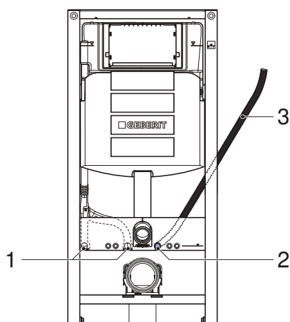
Figura 19: Elemento Geberit Duofix per vaso sospeso con tubo foderato vuoto per allacciamento elettrico
