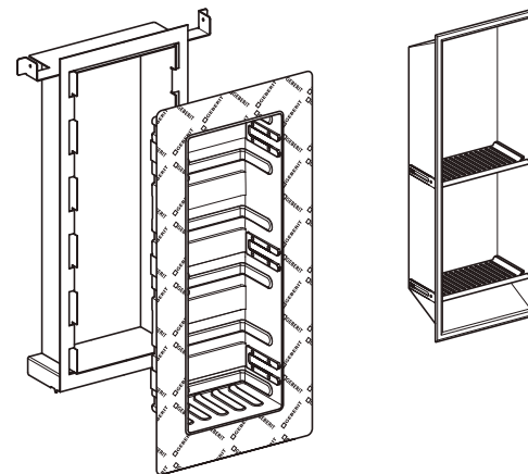
Figura 13: Modulo Geberit Duofix per nicchia portaoggetti con ripiani e Nicchia portaoggetti con ripiani
