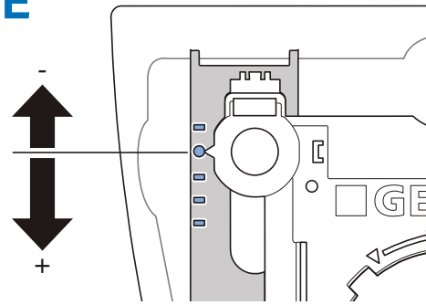
Figura 8: Regolazione dell'altezza (+3 cm/-1 cm) sul vaso sospeso Geberit ONE
