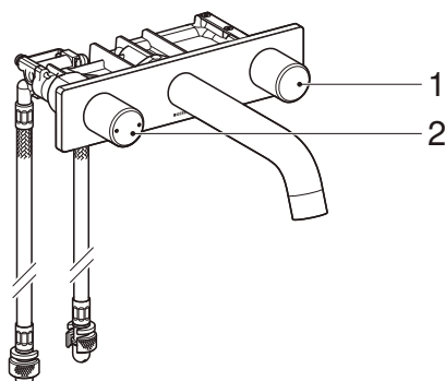
Figura 3: Rubinetteria, design arrotondato, montaggio a parete, miscelatore a due manopole, per vano sifone da incasso
