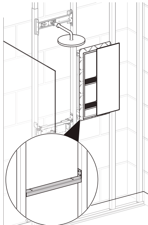
Figura 21: Variante di installazione nicchia portaoggetti con ripiani con barra di fissaggio
