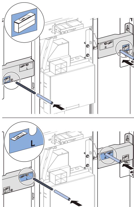
Figura 16: Posizione di montaggio delle barre filettate sull'elemento d'installazione per alloggiamento lavabo
