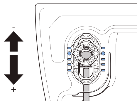
Figura 10: Regolazione dell'altezza (+3 cm/-1 cm) sul bidet sospeso Geberit ONE
