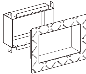
Figura 12: Modulo Geberit Duofix per nicchia portaoggetti rivestibile con piastrelle
