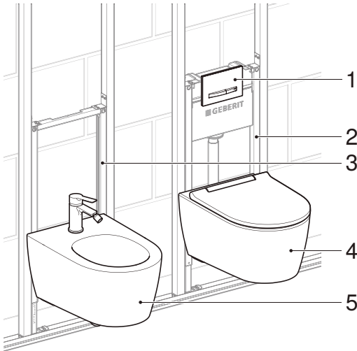
Figura 7: Zona sanitari con Geberit ONE in parete leggera con Geberit Duofix
