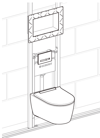
Figura 20: Variante di installazione sopra il vaso con modulo Geberit Duofix per nicchia portaoggetti rivestibile con piastrelle
