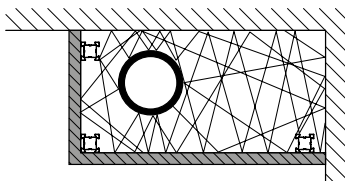
← Riflessione sonora nel vano tecnico senza rivestimento fonoassorbente.
