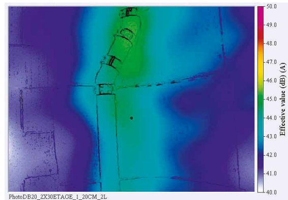
↑ Colonna di scarico con due braghe a 30° in media +7 dB(A)
