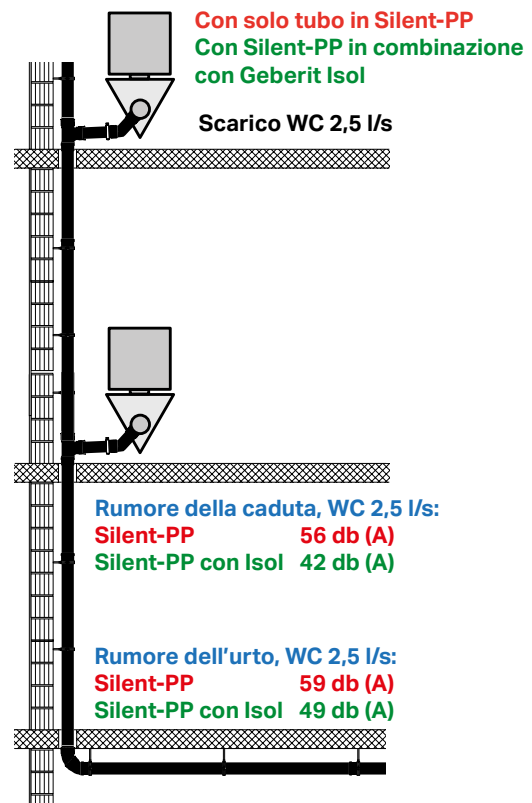
↓ Valori in dB(A) misurati nei laboratori Geberit.
