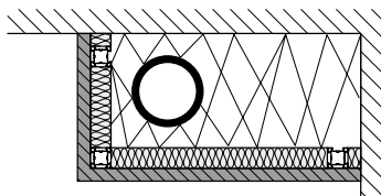
← Riflessione sonora nel vano tecnico con rivestimento fonoassorbente.
