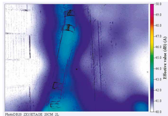
↑ Colonna di scarico con due braghe a 15° in media +5 dB(A)
