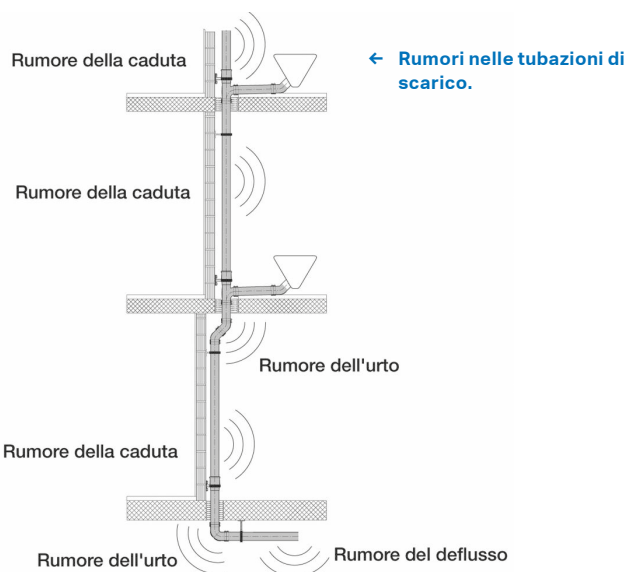
↑ Colonna di scarico con due braghe a 30° in media +7 dB(A)
