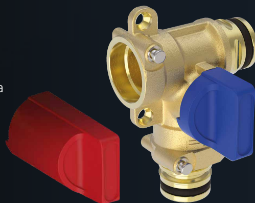
↑ Set valvola a T con manopola blu o rossa intercambiabile a scelta.
